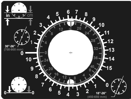
DEPTH INDICATOR P/N 191752 (18"-36") P/N 198018 (48" Blade) P/N 198062 (60" Blade)
