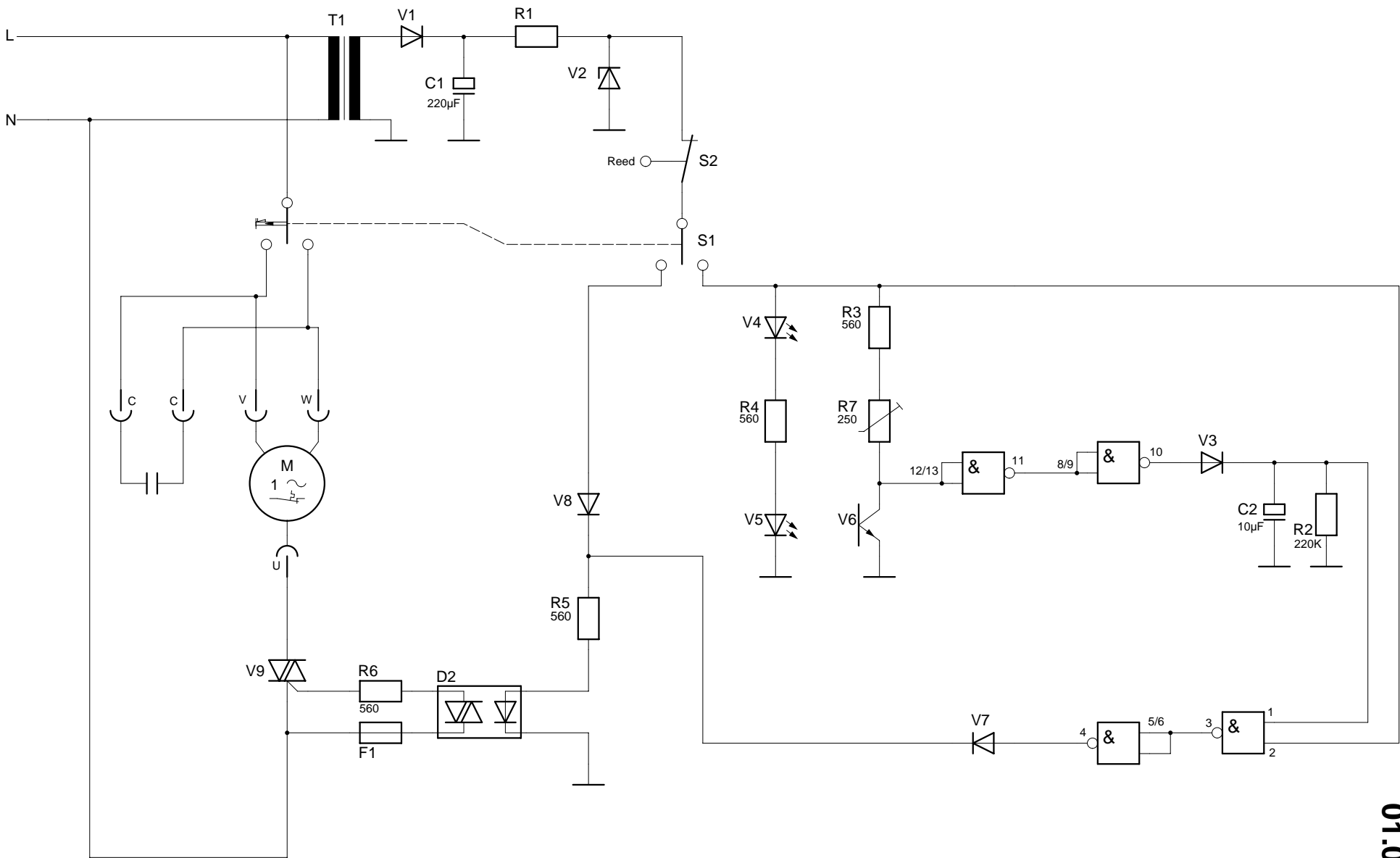
Stromlaufplan 2260 A CROSS/CUT schema de circuit électrique 2260 A CROSS/CUT wiring diagram 2260 A CROSS/CUT
