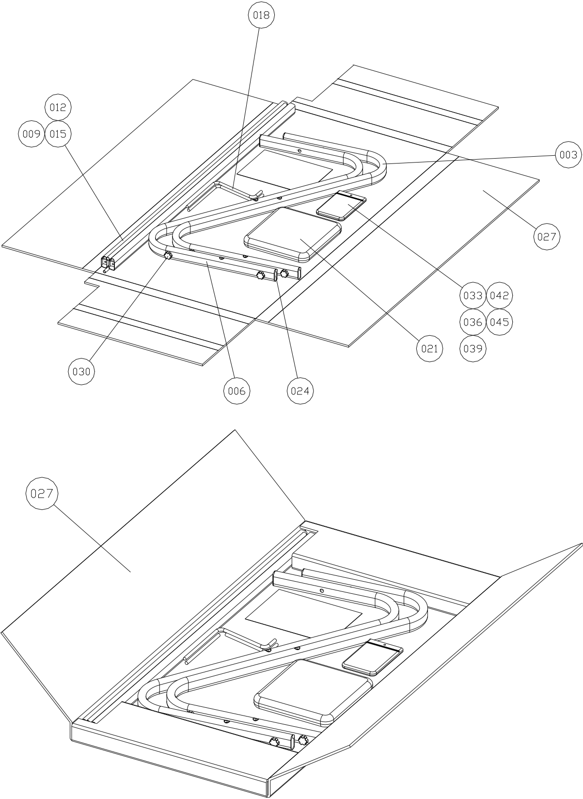
Disegno/Drawing : Dis-012
