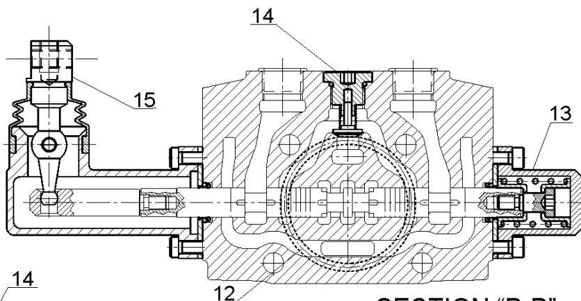
SECTION "B-B" SEZIONE "B-B"
