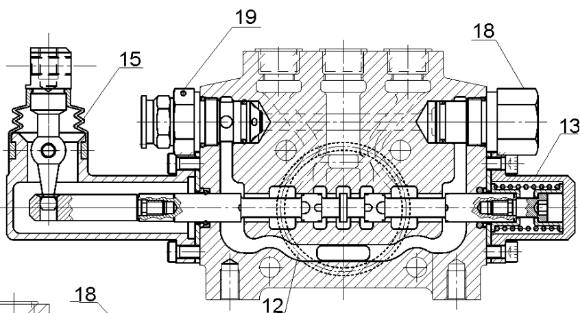
SECTION "D-D" SEZIONE "D-D"
