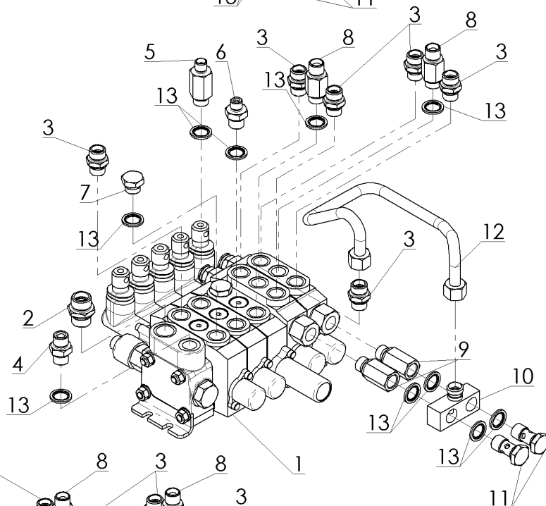
"PLUS" MACHINE (5 ELEMENTS) MACCHINA "PLUS" (5 ELEMENTI)
