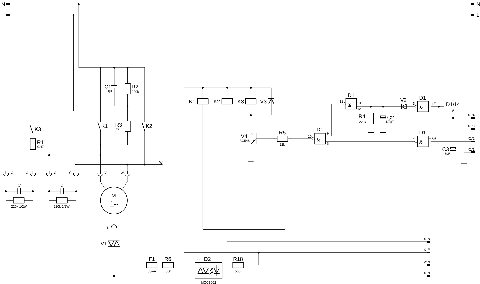
Stromlaufplan 4002 B schema de circuit électrique 4002 B wiring diagram 4002 B
