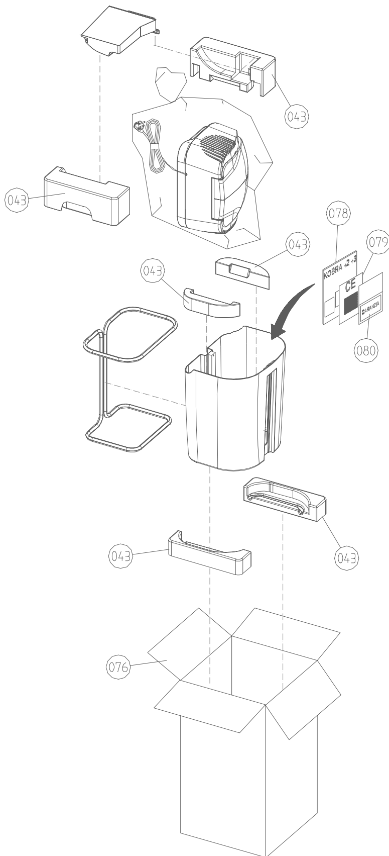
KOBRA +2 S4 / +2 S7 DISEGNO / DRAWING : 03
