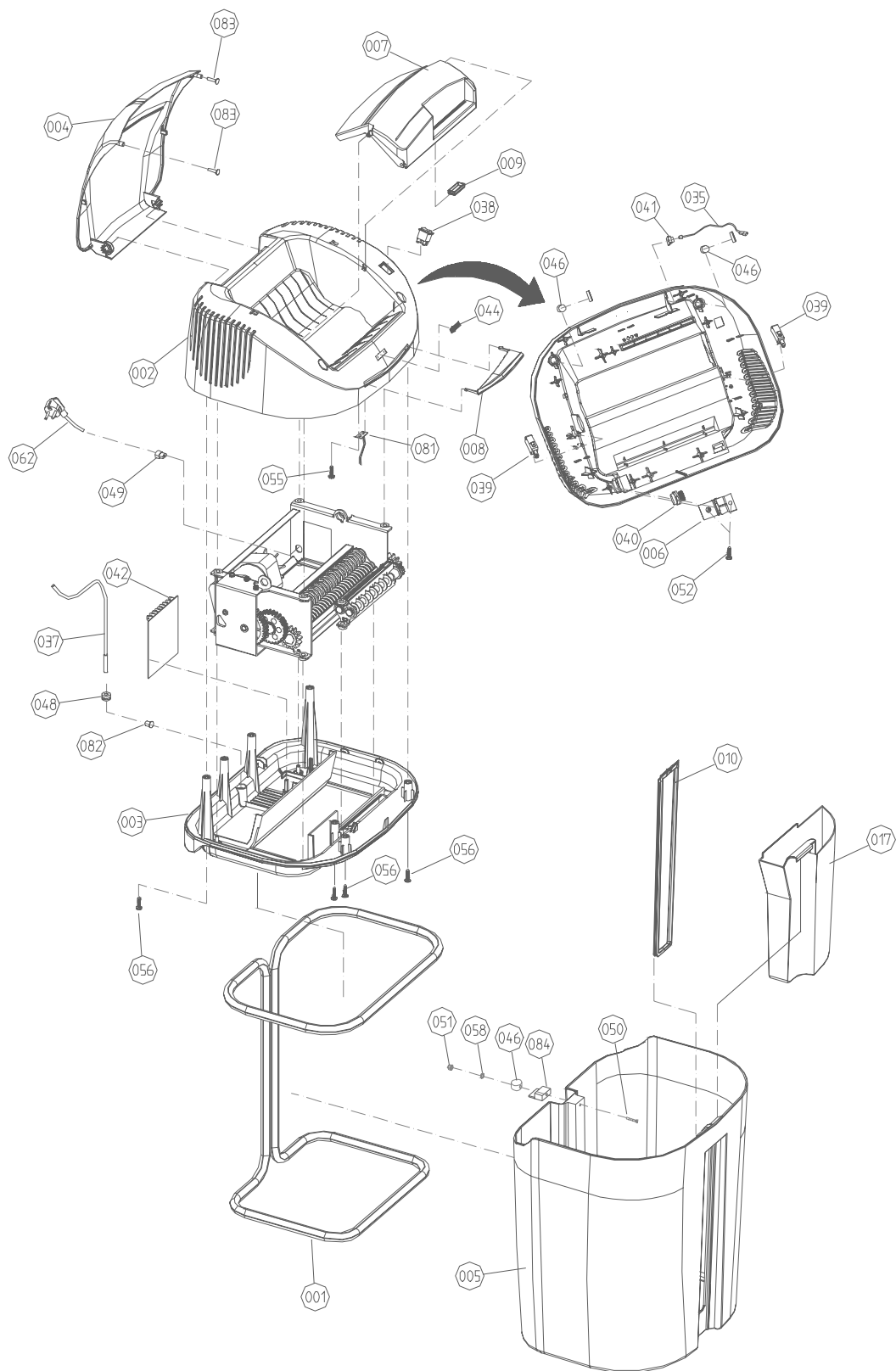
KOBRA +2 S4 / +2 S7 DISEGNO / DRAWING : 01
