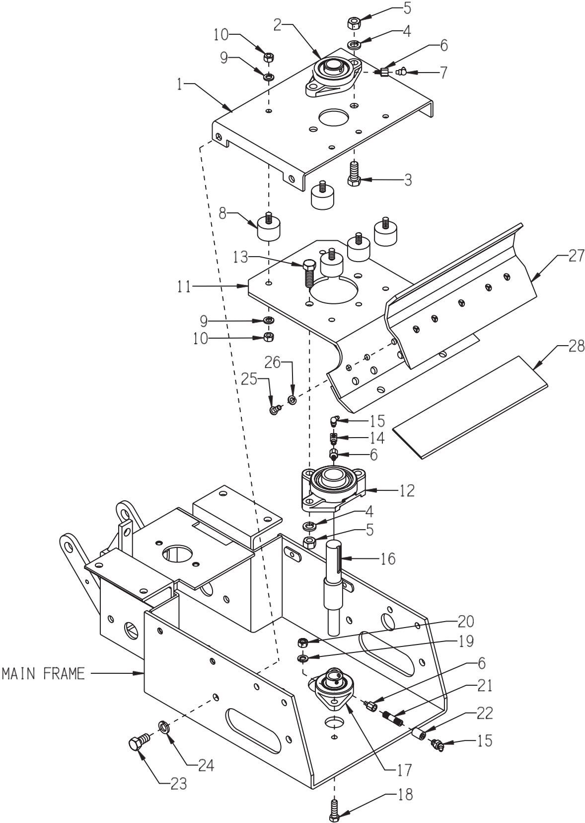
ILLUSTRATION 7 : BLADE & STRIKER PLATE GROUPING
