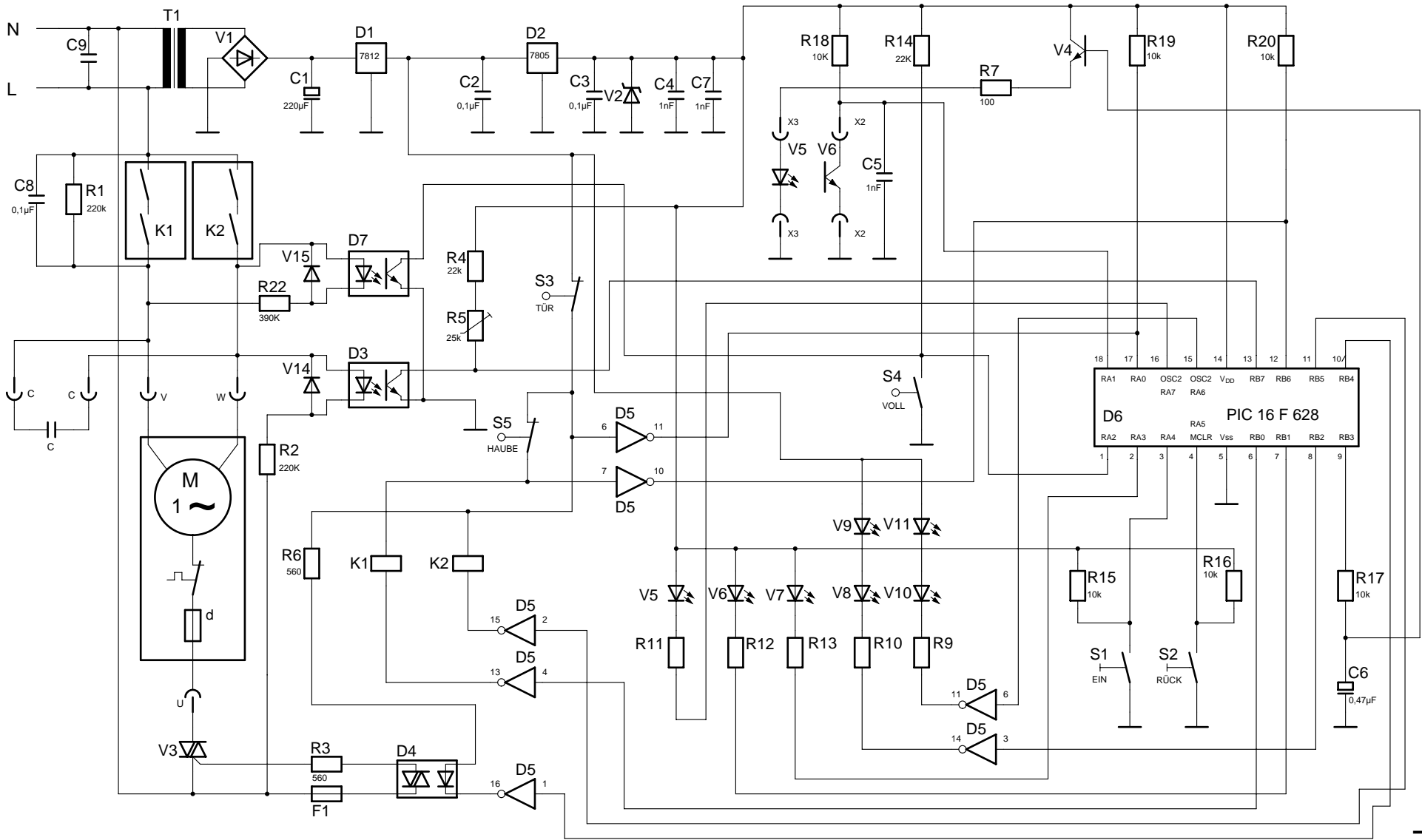
Stromlaufplan 2503 A schema de circuit électrique 2503 A wiring diagram 2503 A
