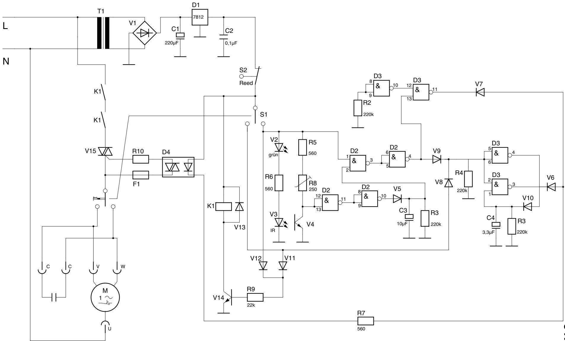
Stromlaufplan 2240 B Cross/Cut schema de circuit électrique 2240 B Cross/Cut wiring diagram 2240 B Cross/Cut
