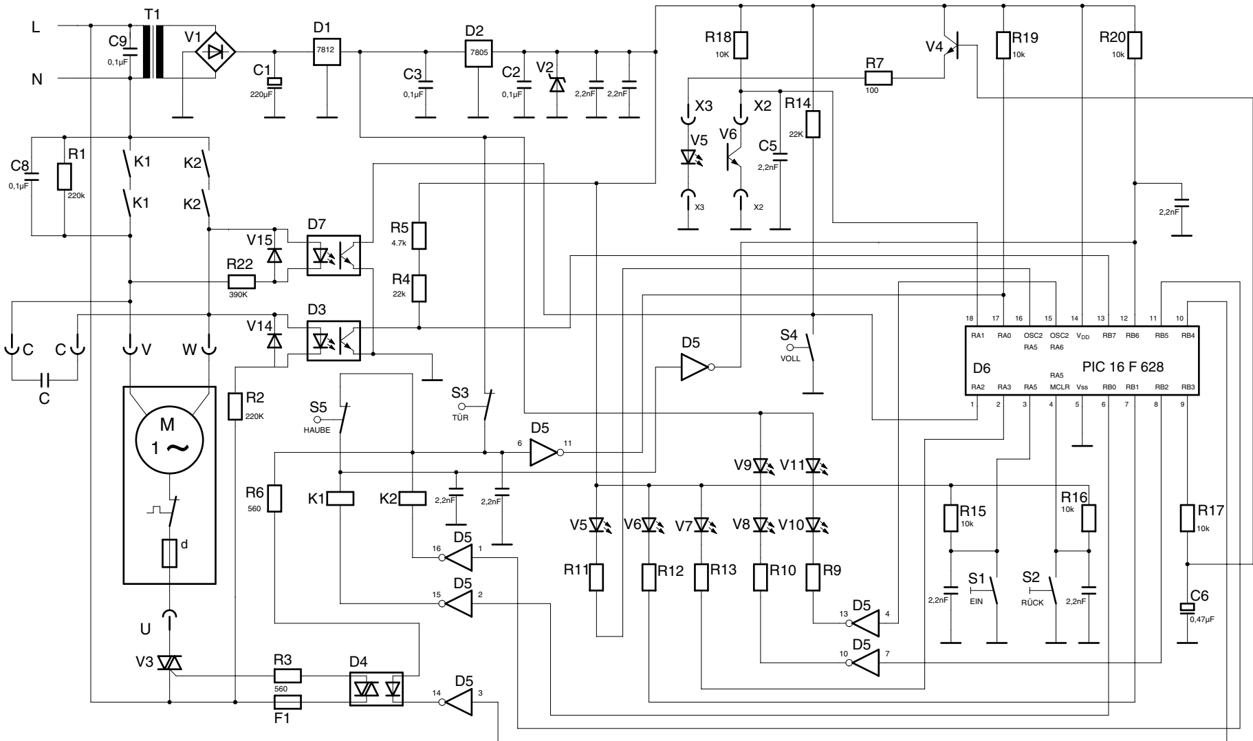
Stromlaufplan 2360 B schema de circuit électrique 2360 B wiring diagram 2360 B
