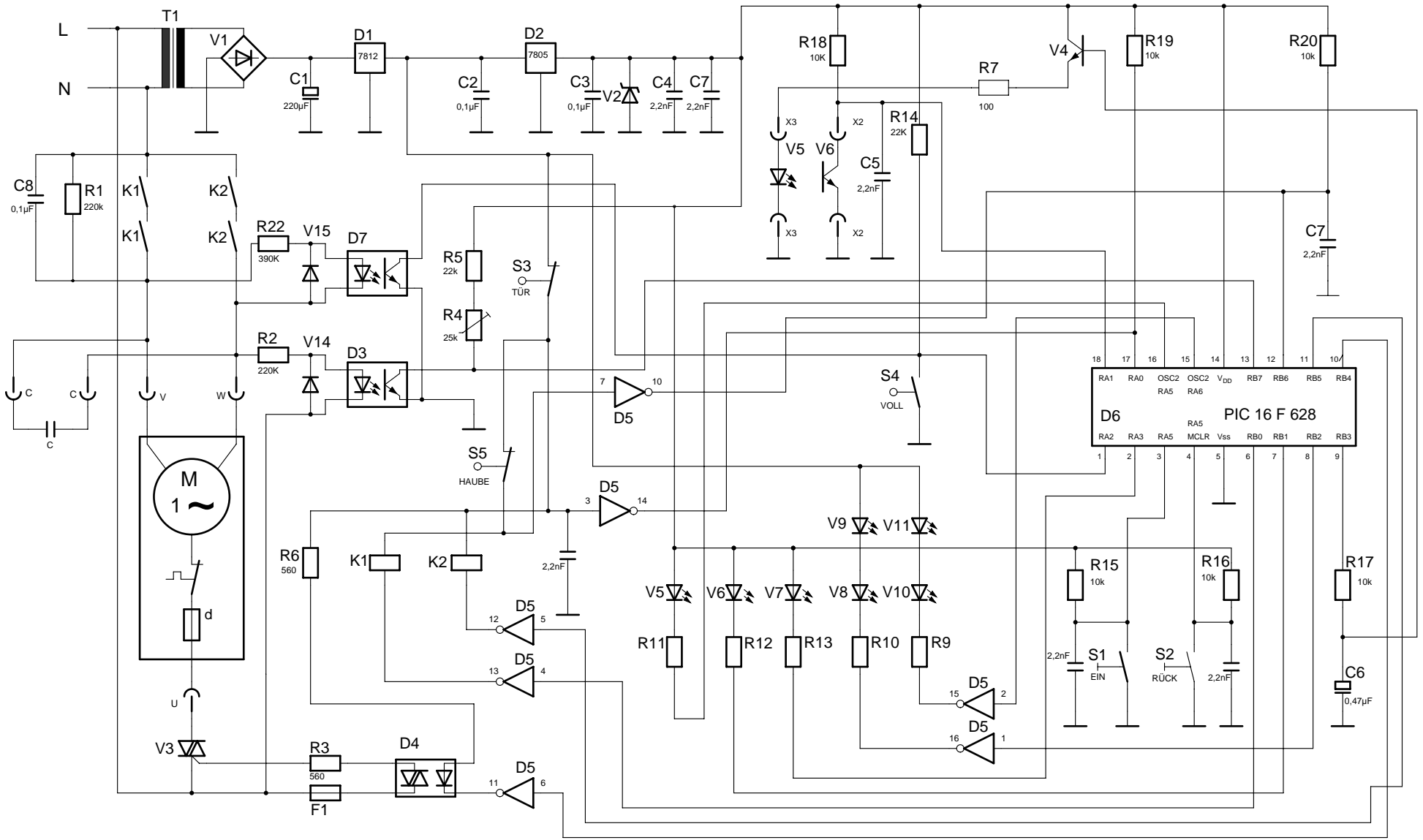
Stromlaufplan 2603 A schema de circuit électrique 2603 A wiring diagram 2603 A
