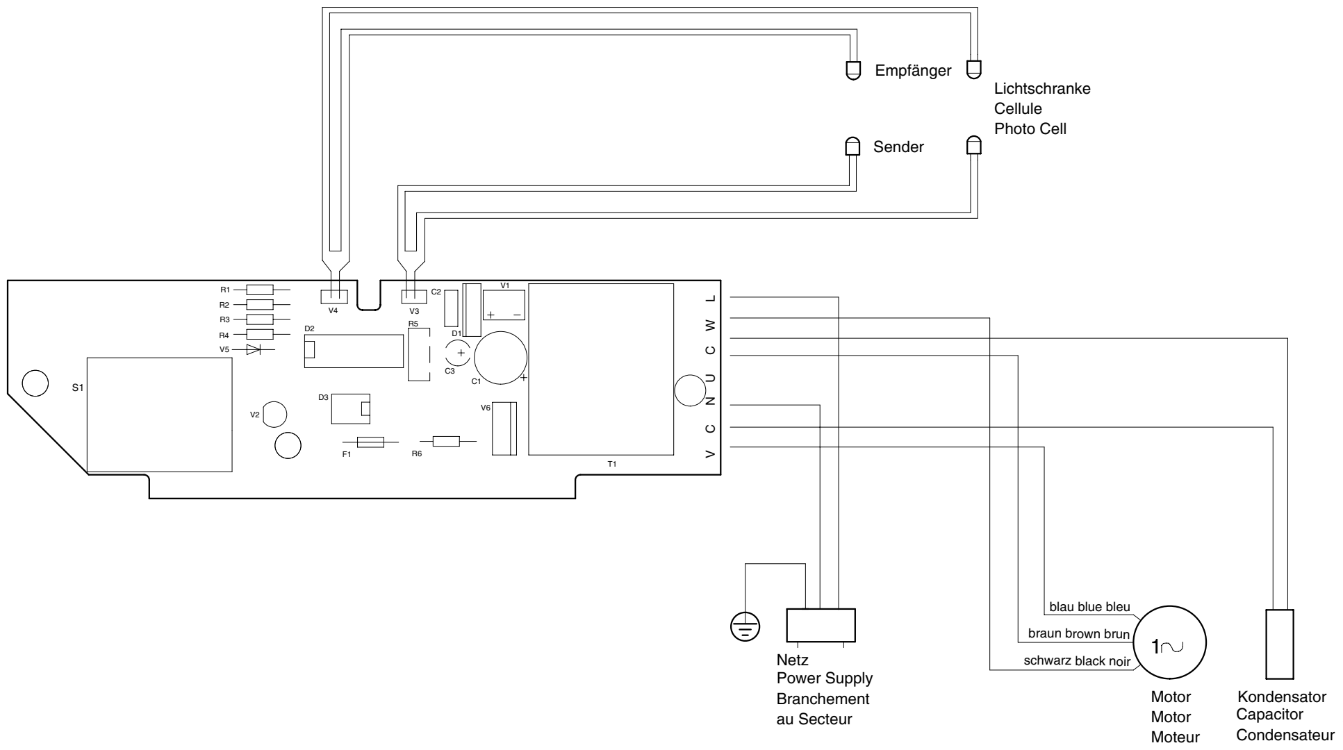
Anschlußplan 2270 B Diagramme de branchement 2270 B Connecting diagram 2270 B
