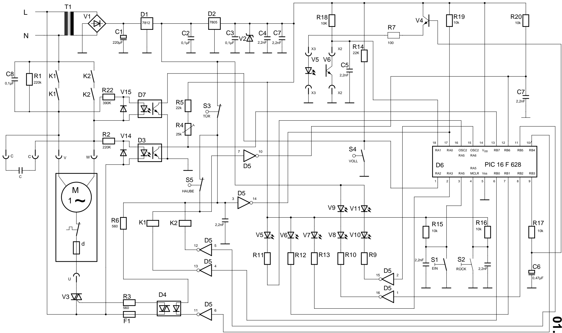
Stromlaufplan 3803 A schema de circuit électrique 3803 A wiring diagram 3803 A
