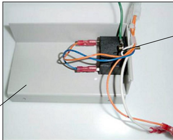
Motor capacitor
