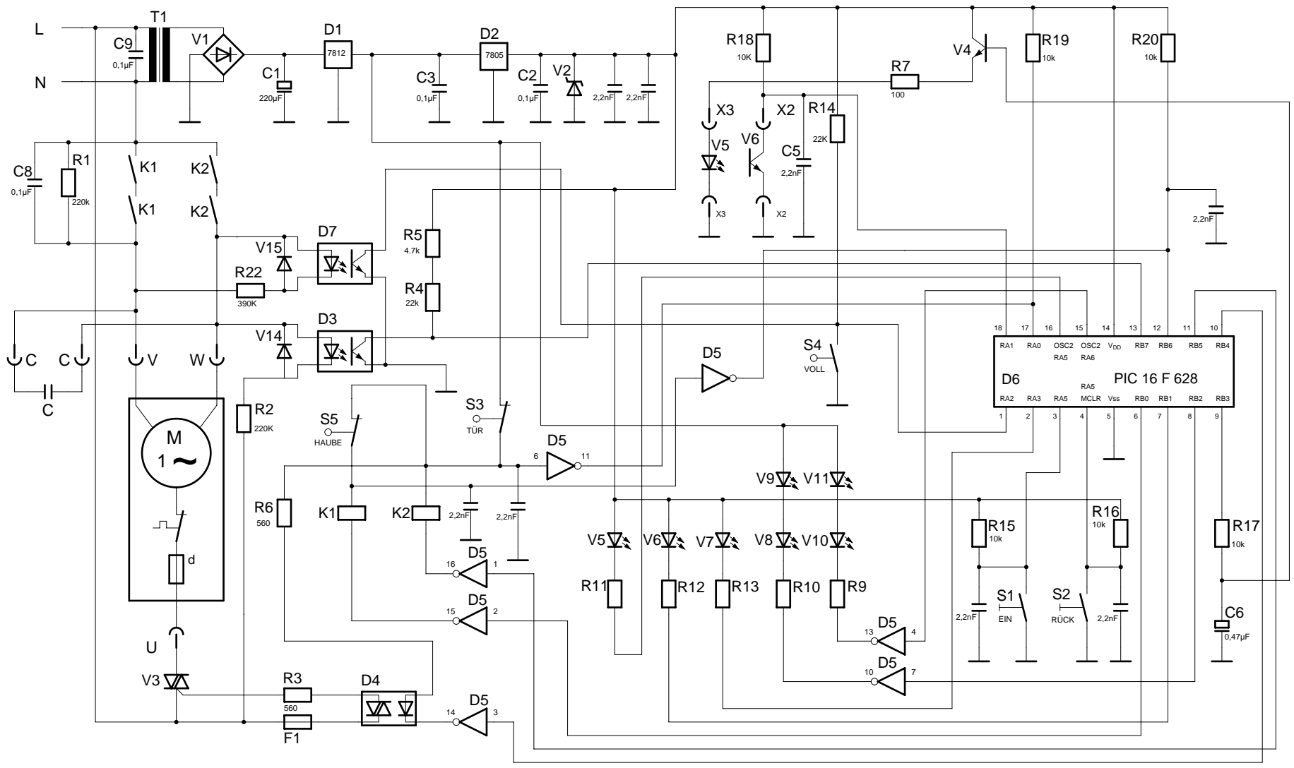
Stromlaufplan 2403 A schema de circuit électrique 2403 A wiring diagram 2403 A
