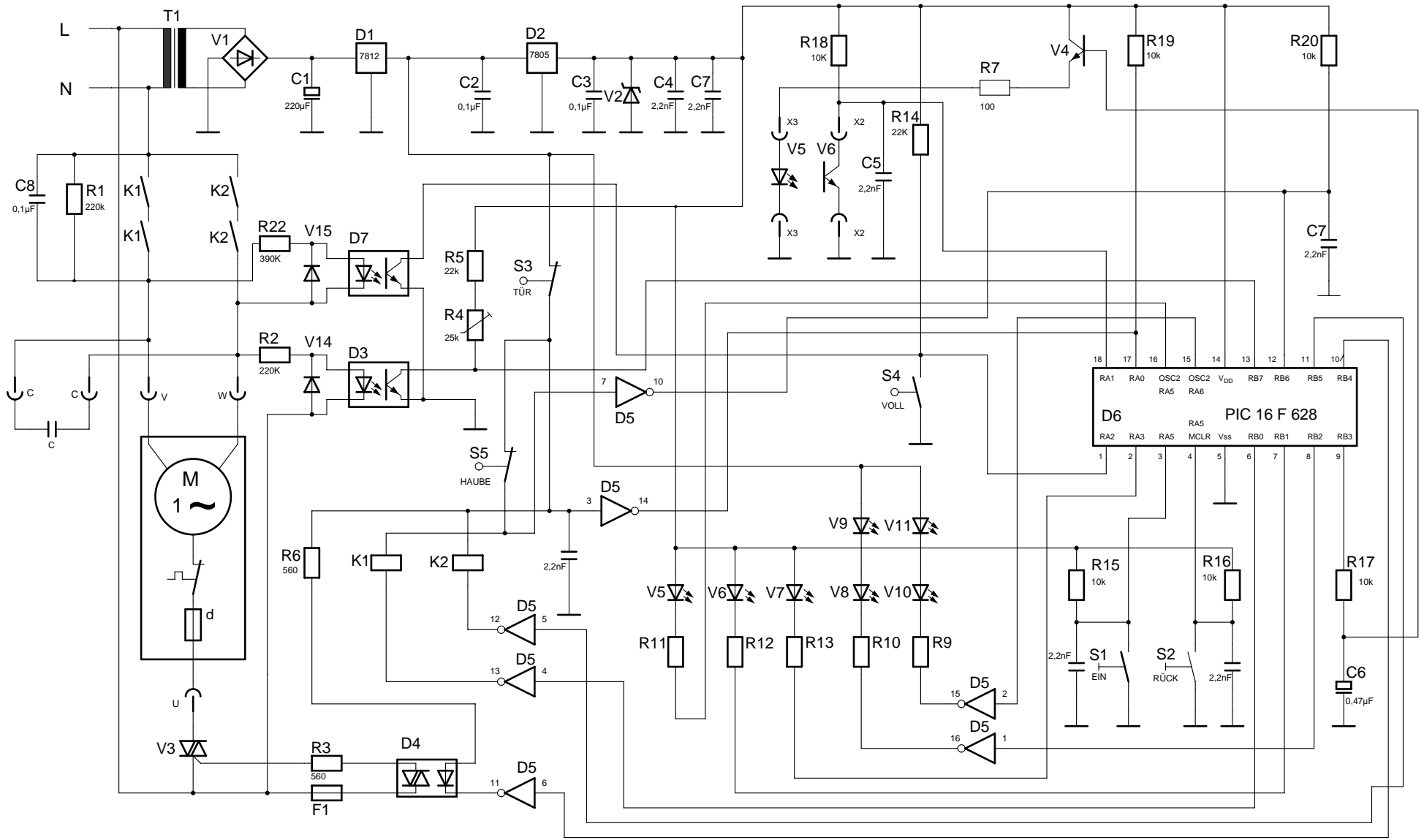
Stromlaufplan 3803 A schema de circuit électrique 3803 A wiring diagram 3803 A
