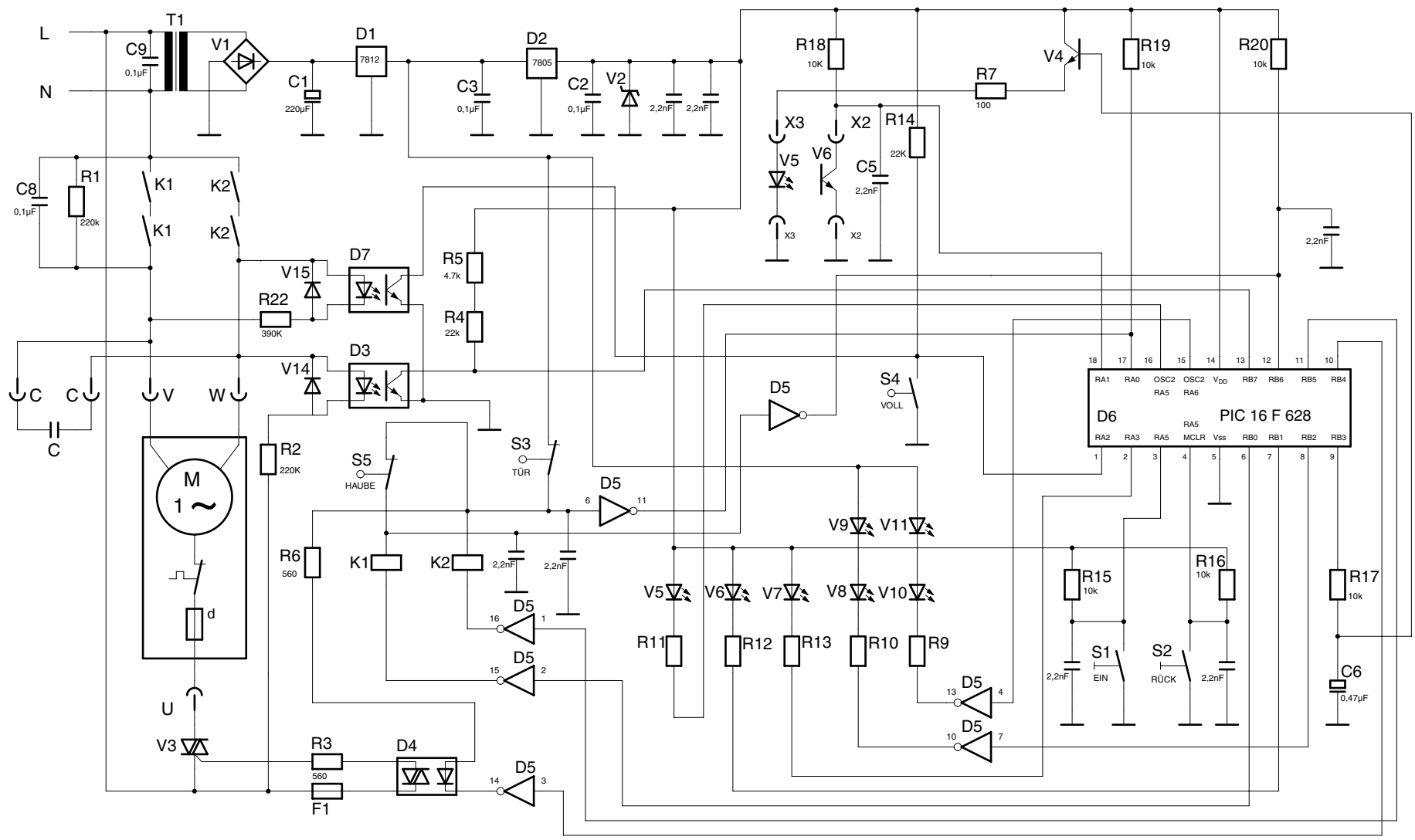
Stromlaufplan 2404 A schema de circuit ectrique 2404 A wiring diagram 2404 A
