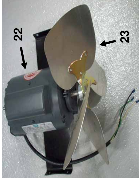
Fan and Motor
