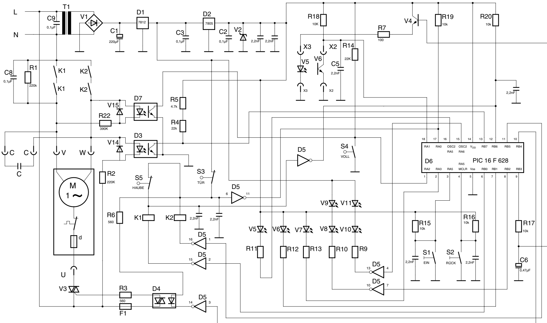
Stromlaufplan 2404 B schema de circuit ectrique 2404 B wiring diagram 2404 B
