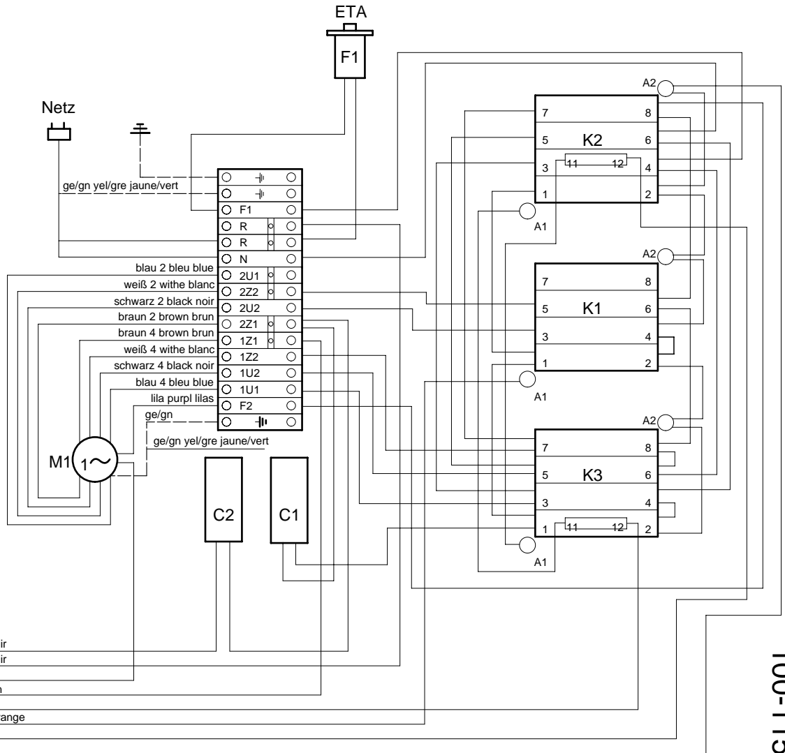
Anschlußplan 4004 E Diagramme de branchement 4004 E Conecting diagram 4004 E
