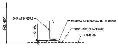
2 DOOR THRESHOLD DETAIL A2 SCALE: N.T.S.
