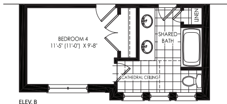
ELEV. B
