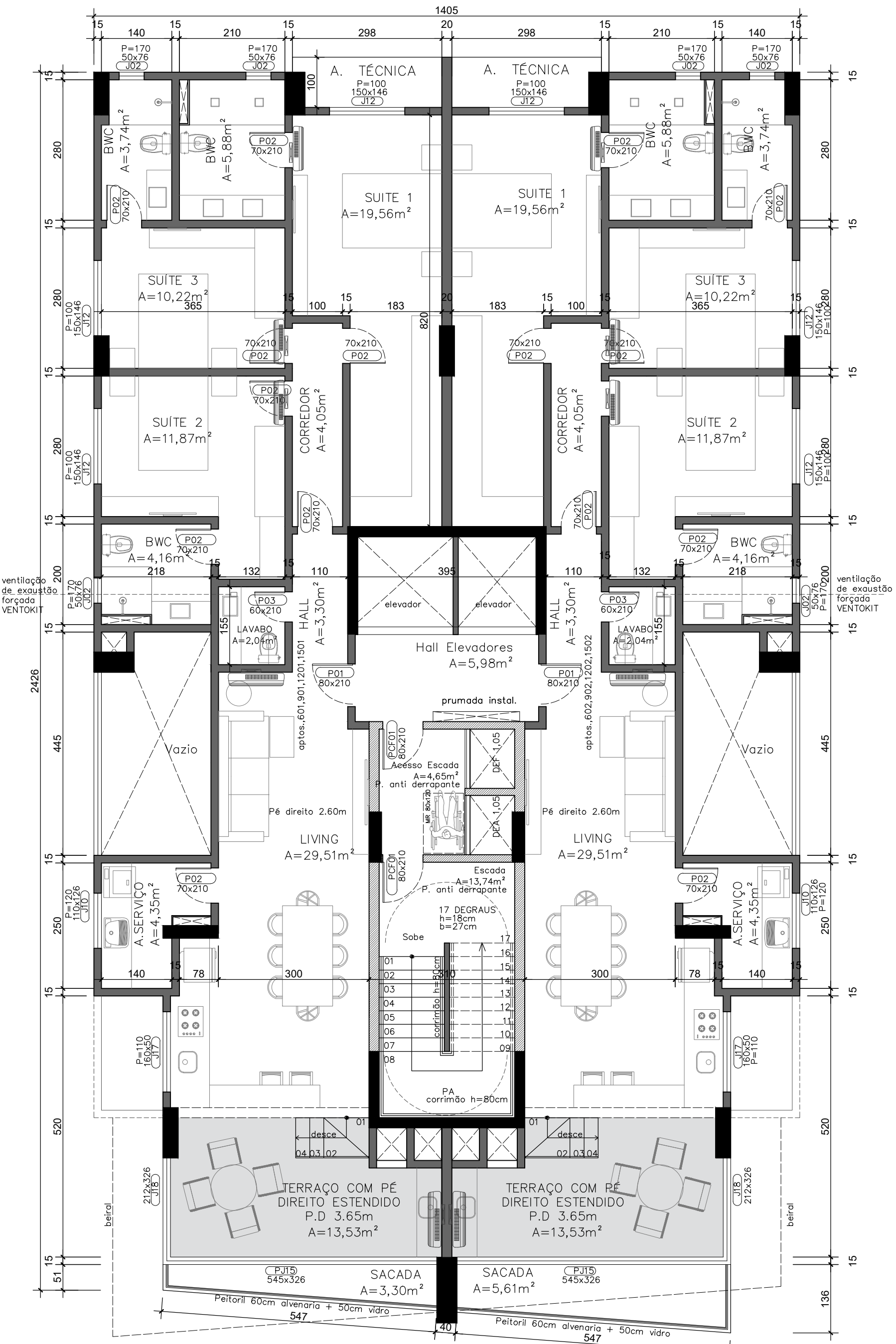
TIPO 03 FINAL 01 A=137,06m 2
